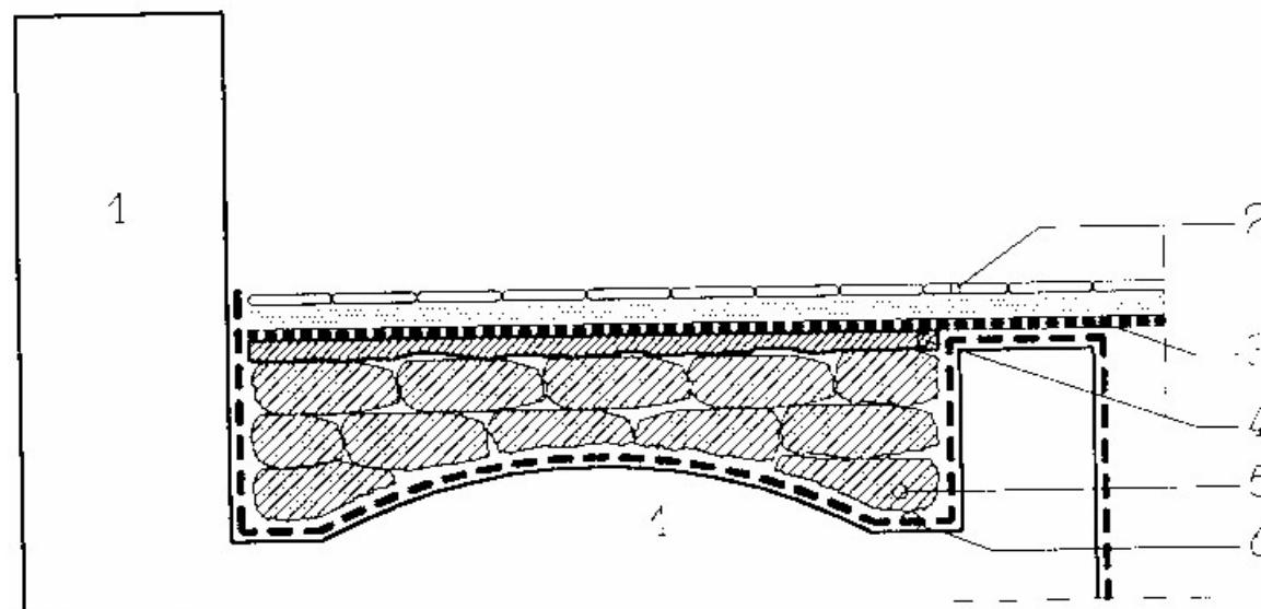
Εικόνα 2 Σχέδιο πλακόστρωσης. Α. Υπάρχουσα λιθοδομή. Β. Πλακόστρωτο. Γ. Ασφαλτόπανο με ψηφίδες. Δ. Τσιμεντοκονίαμα εξομάλυνσης 5 εκ. Πλέγμα ή ίνες Ε. Χονδρό νάιλον
